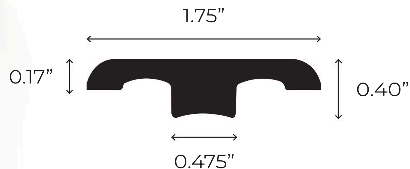
T-MOLDING
