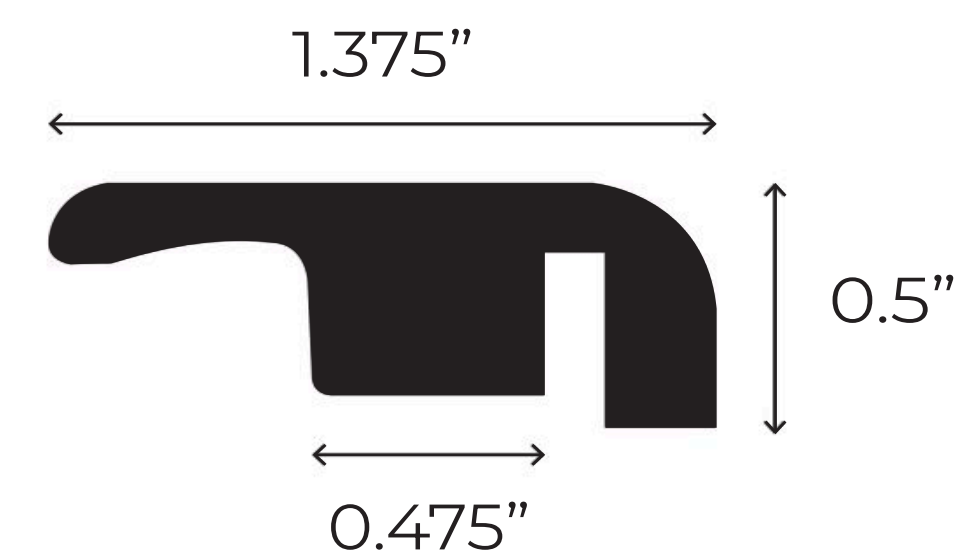
END CAP
